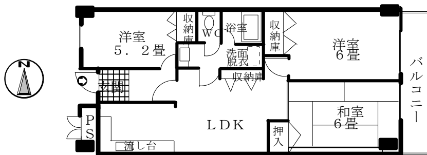
エスポアール石橋平面図
